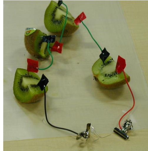
レモン電池
